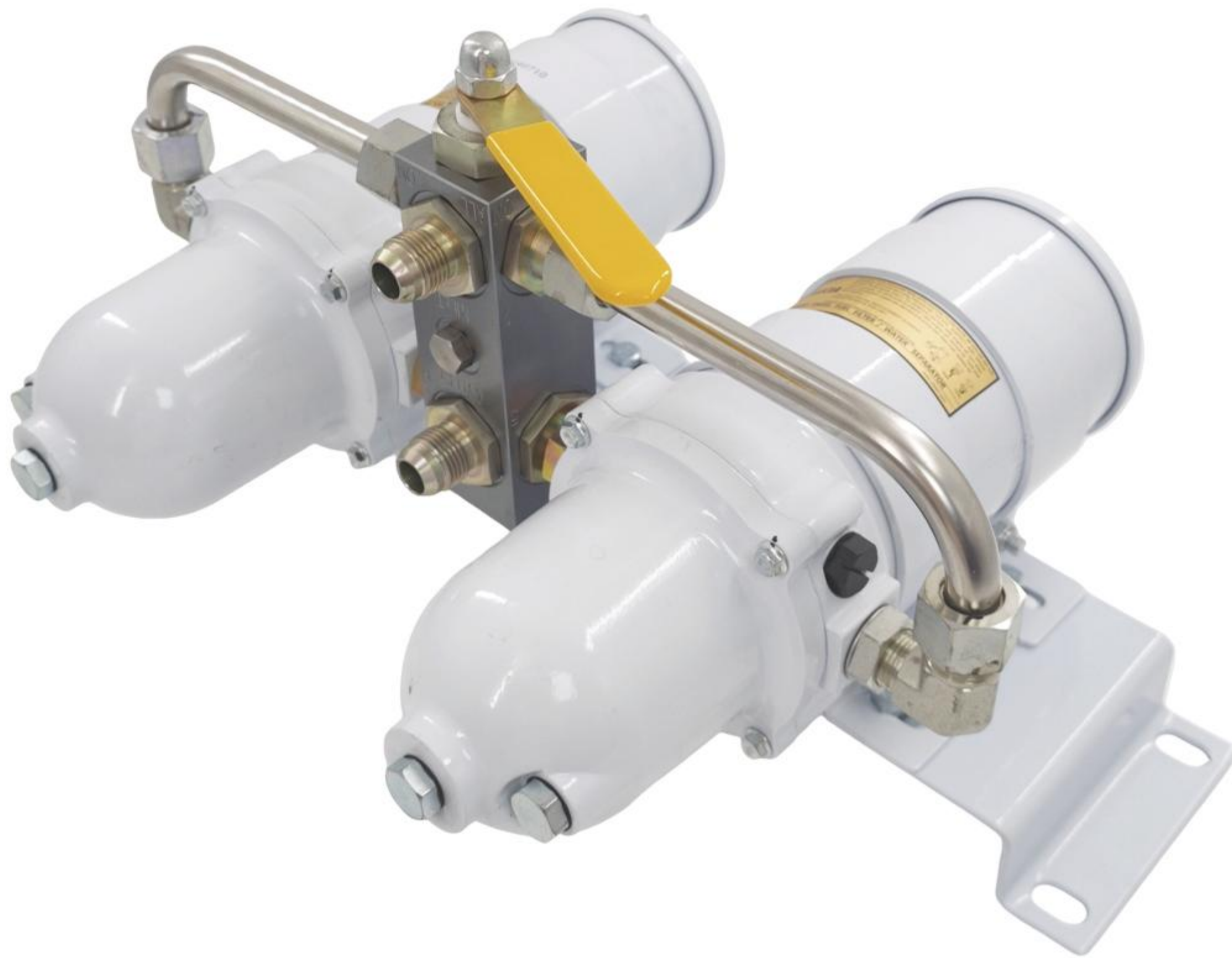
FWS341-DL( 双联 )
